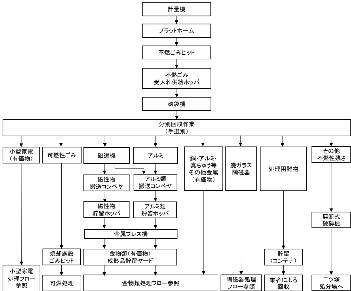
図 2-6 ① もやせないごみの処理フロー
