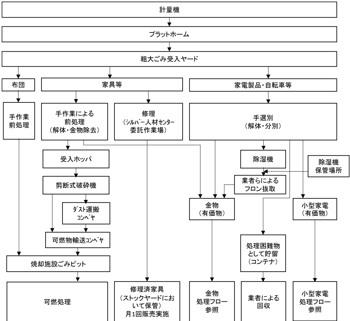
図 2-6② 粗大ごみの処理フロー
