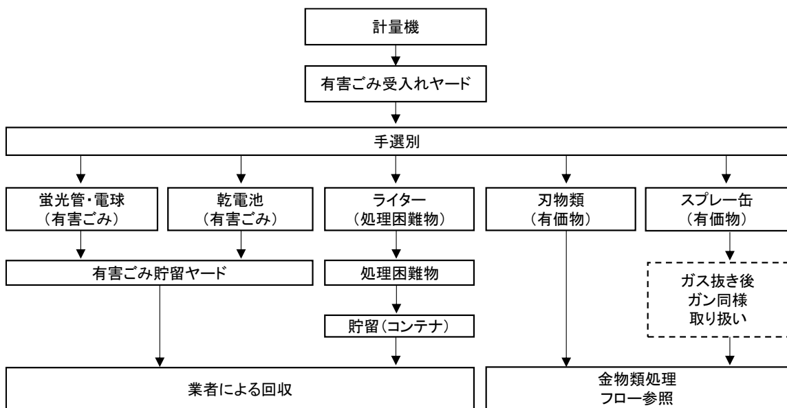
図 2-6③ 有害ごみの処理フロー
