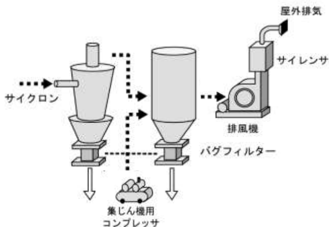
図4-11 サイクロン+バグフィルタのイメージ図
