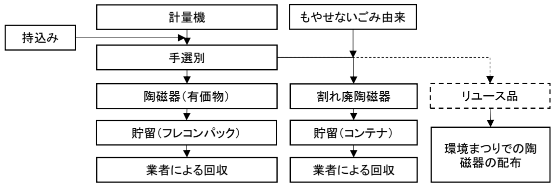
図 2-6 ⑩ 陶磁器の処理フロー
