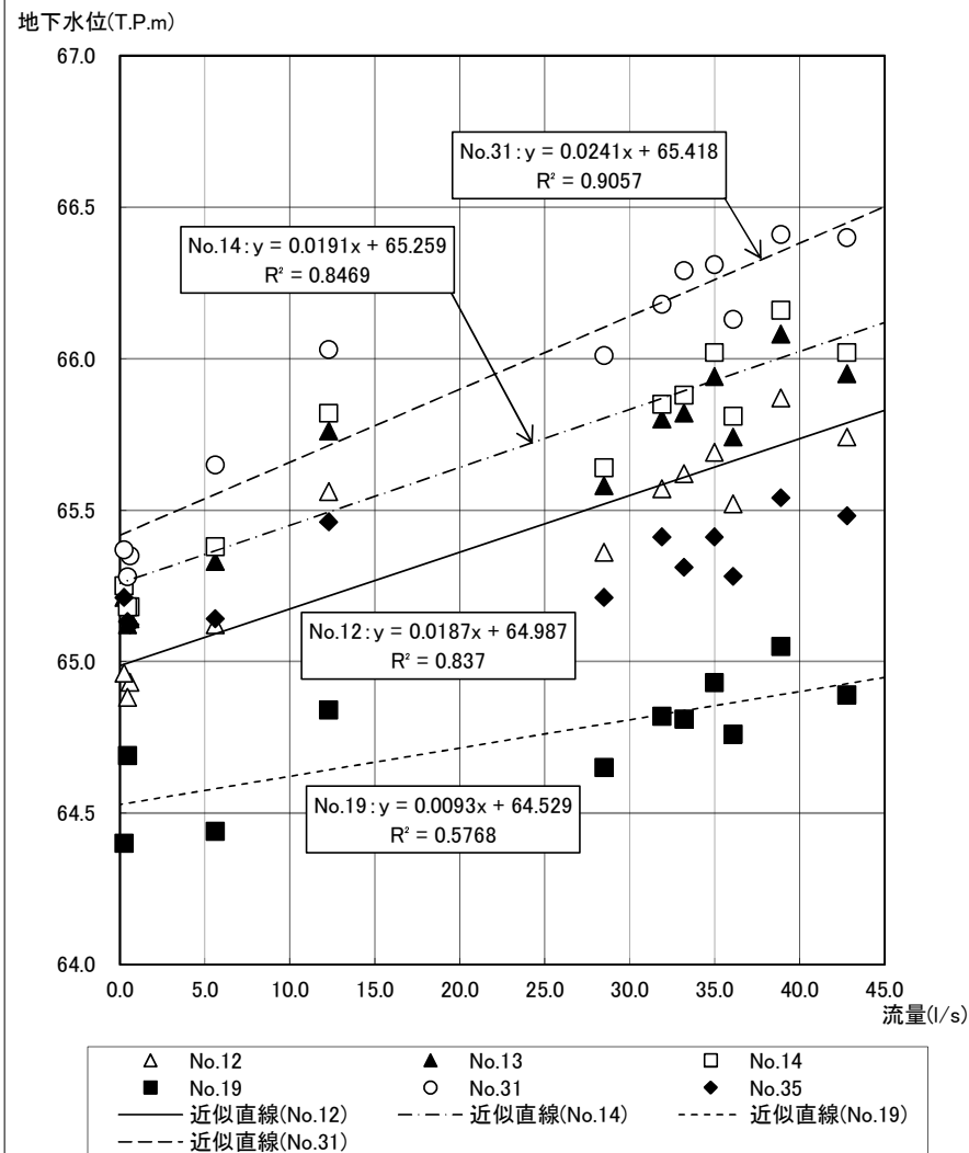
図-3.3(2) 主要湧水の湧水量と地下水位の関係 (2/3)
