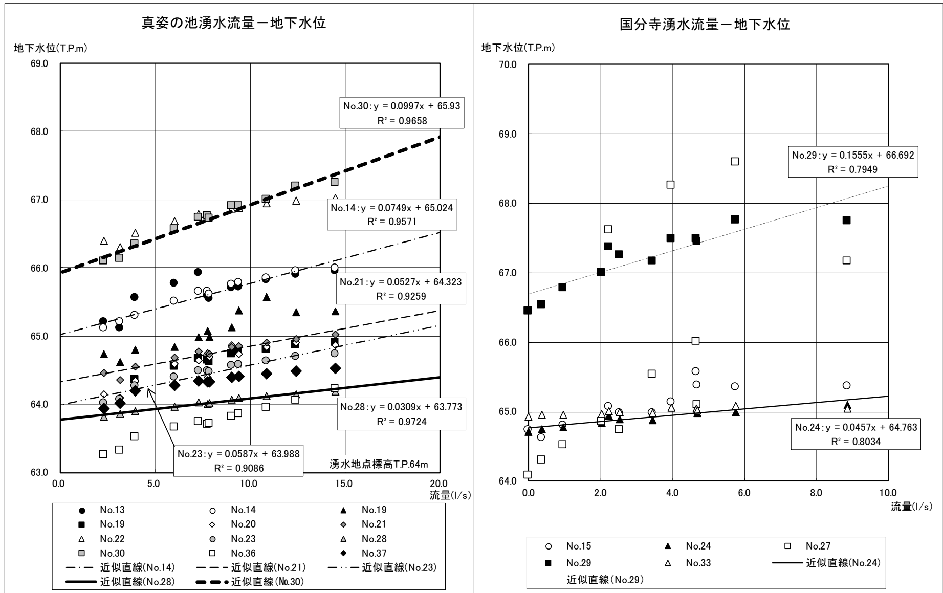
図-3.3(1) 主要湧水の湧水量と地下水位の関係(1/3)
