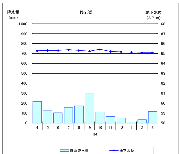
図-3.2(5) 地下水位測定結果及び気象庁府中観測所雨量 (5//7)
