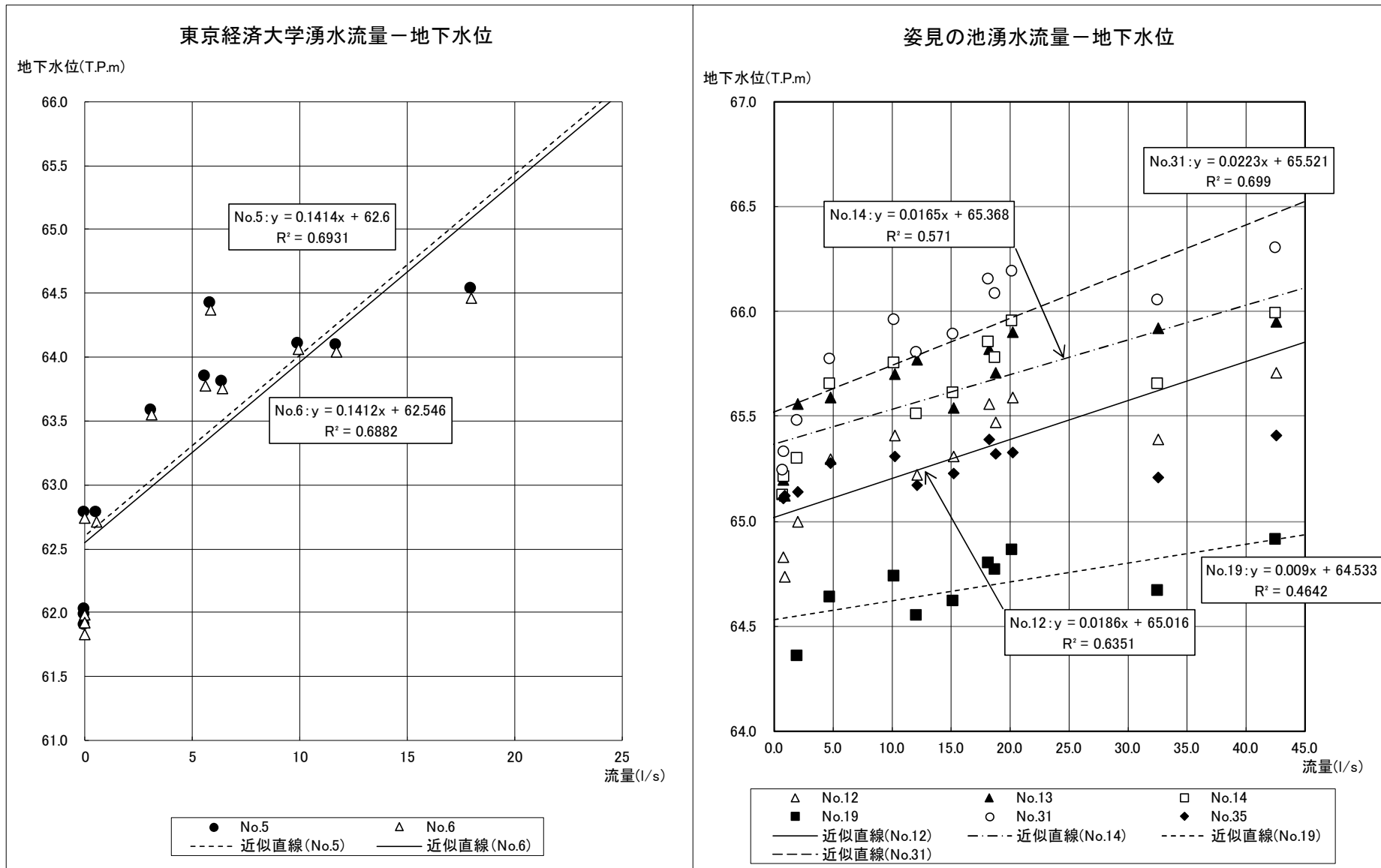
図-3.3(2) 主要湧水の湧水量と地下水位の関係(2/3)
