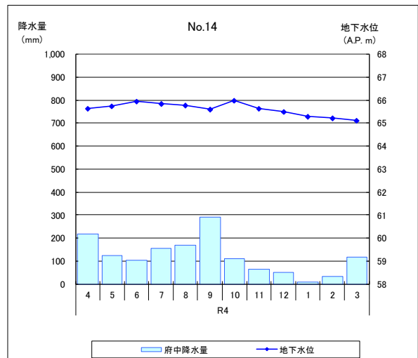
図-3.2(2) 地下水位測定結果及び気象庁府中観測所雨量 (2//7)
