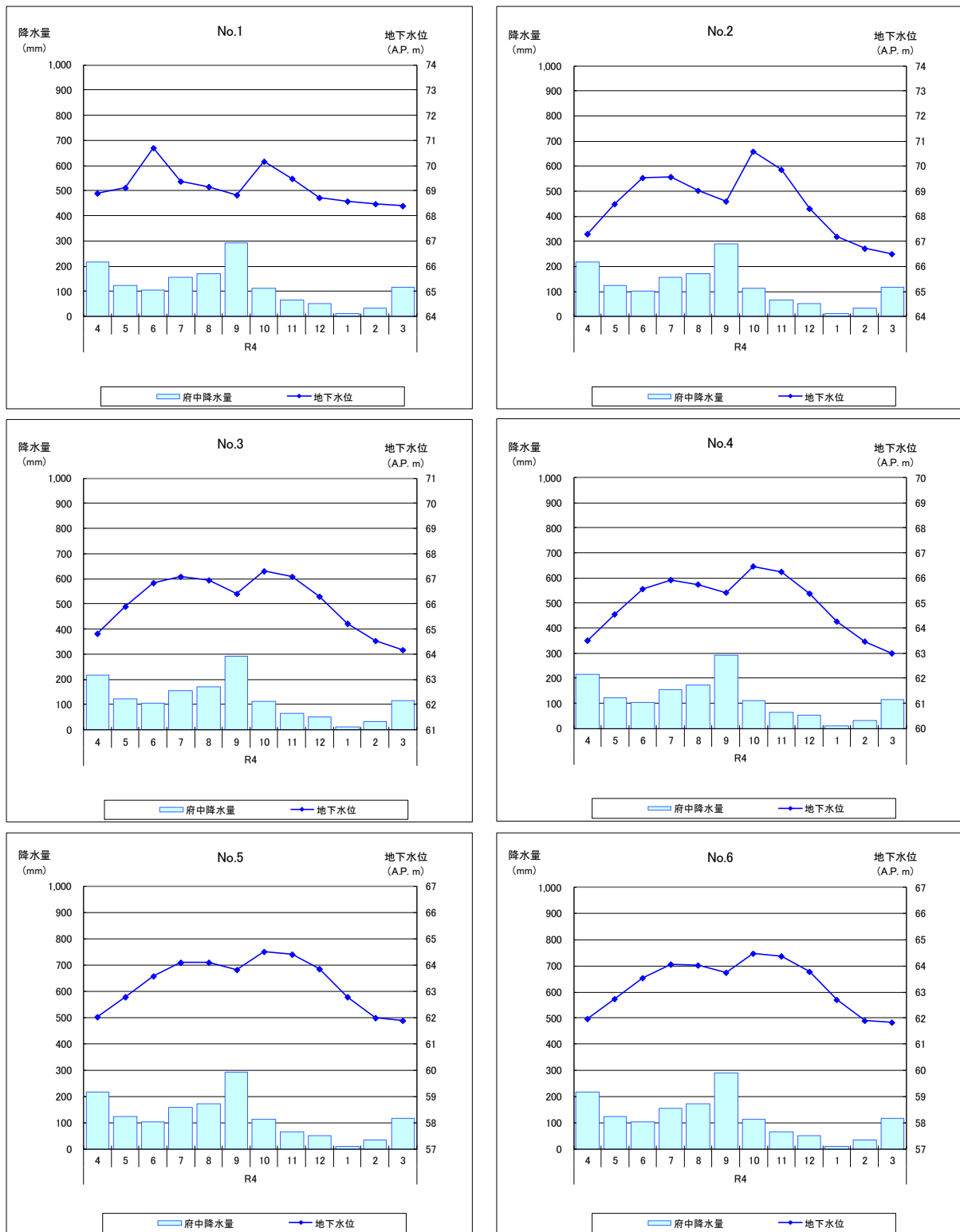
図-3.2(1) 地下水位測定結果及び気象庁府中観測所雨量 (1//7)
