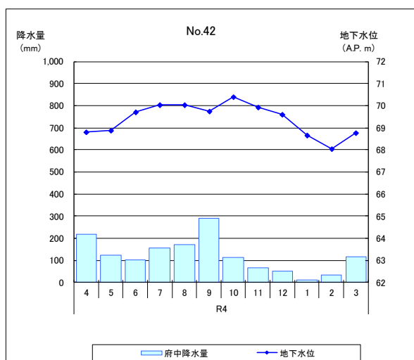
図-3.2(7) 地下水位測定結果及び気象庁府中観測所雨量 (7/7)
