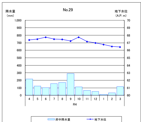
図-3.2(4) 地下水位測定結果及び気象庁府中観測所雨量 (4//7)
