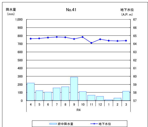
図-3.2(6) 地下水位測定結果及び気象庁府中観測所雨量 (6//7)
