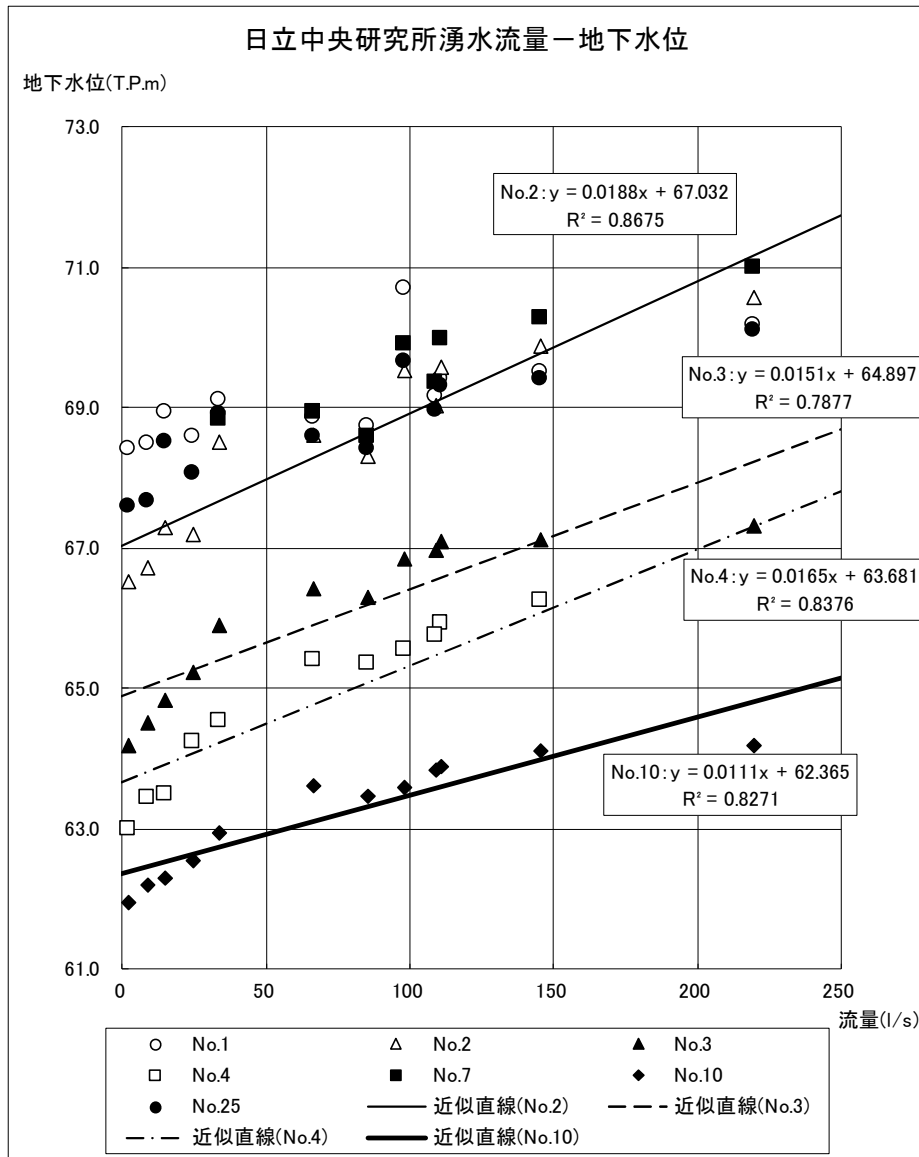
図-3.3(3) 主要湧水の湧水量と地下水位の関係(3/3)
