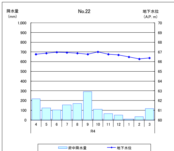
図-3.2(3) 地下水位測定結果及び気象庁府中観測所雨量 (3//7)
