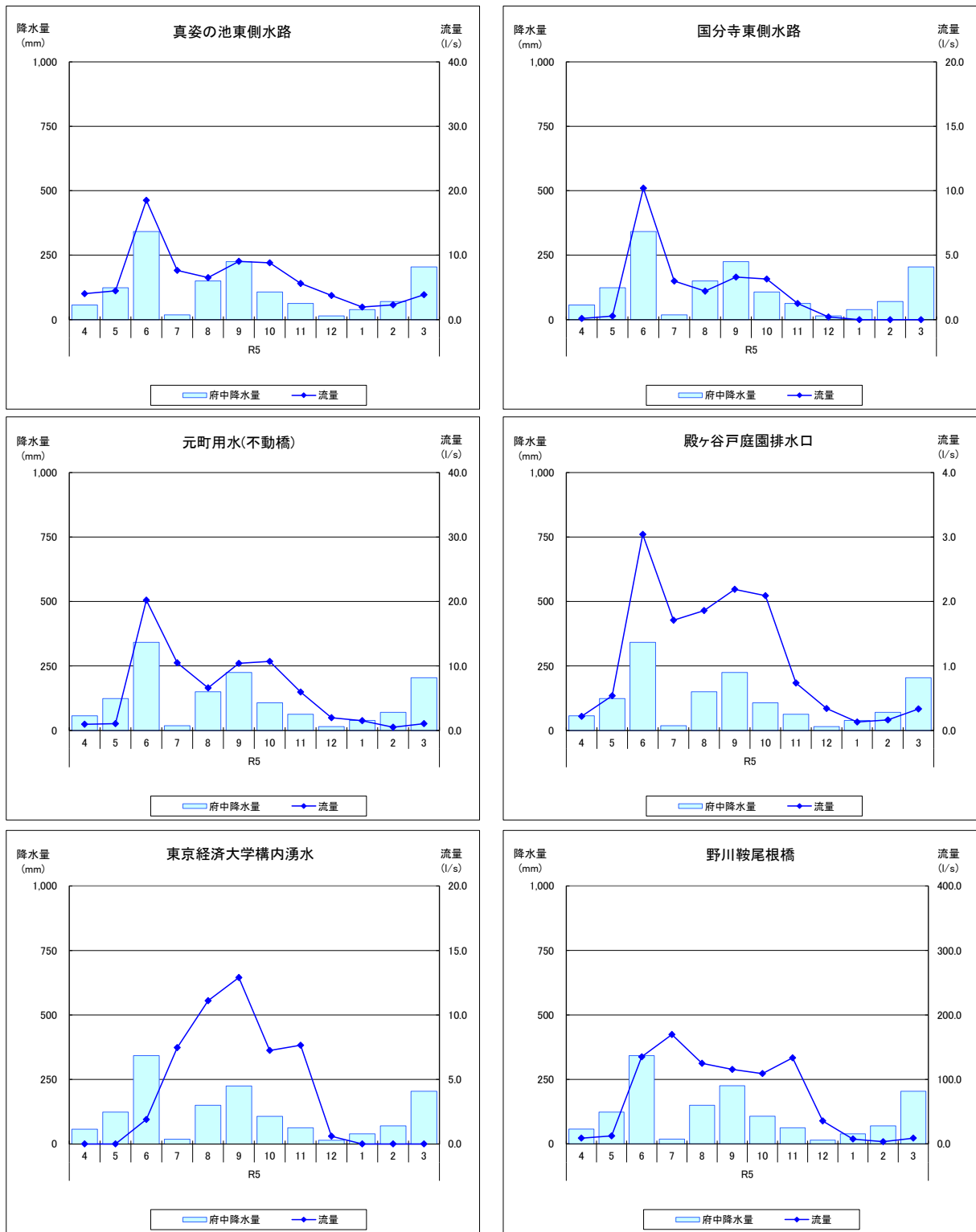
図-3.1(1) 流量測定結果及び気象庁府中観測所雨量 (1/2)
