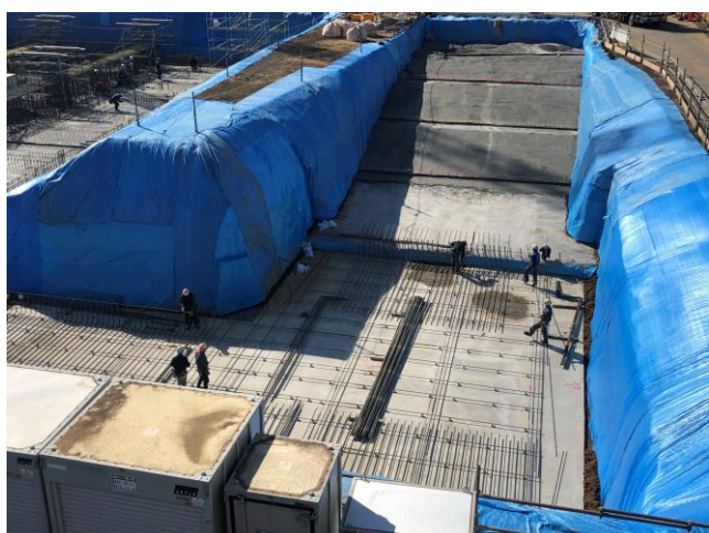
スロープ部基礎配筋 (2/15)
