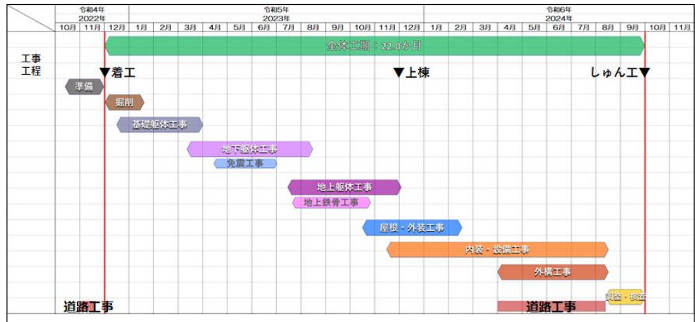
工事工程表
