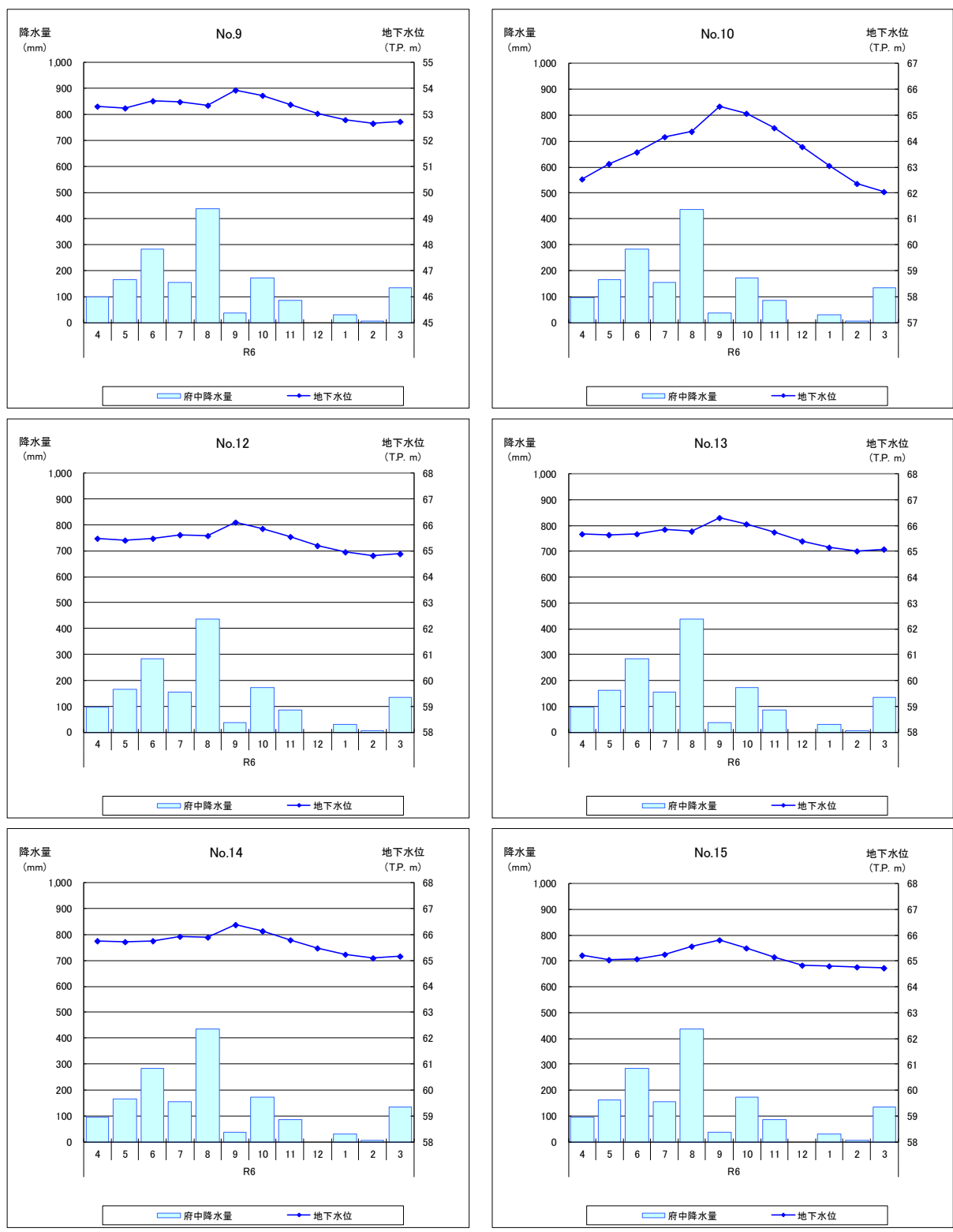
図-3.2(2) 地下水位測定結果及び気象庁府中観測所雨量 (2/6)
