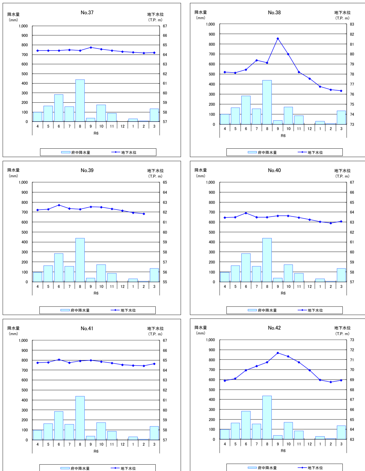
図-3.2(6) 地下水位測定結果及び気象庁府中観測所雨量 (6/6)
