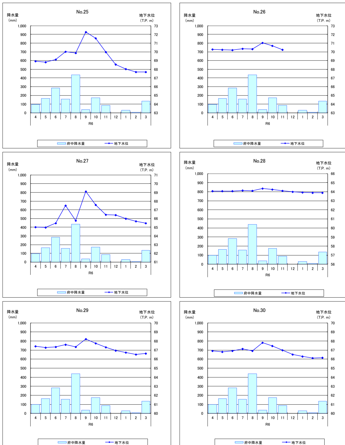
図-3.2(4) 地下水位測定結果及び気象庁府中観測所雨量 (4/6)
