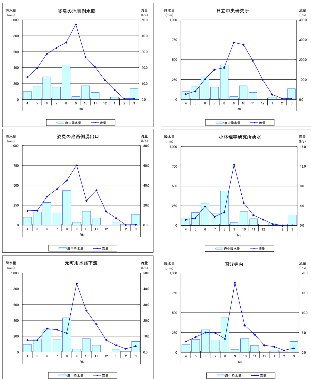
図-3.1(2) 流量測定結果及び気象庁府中観測所雨量 (2/2)
