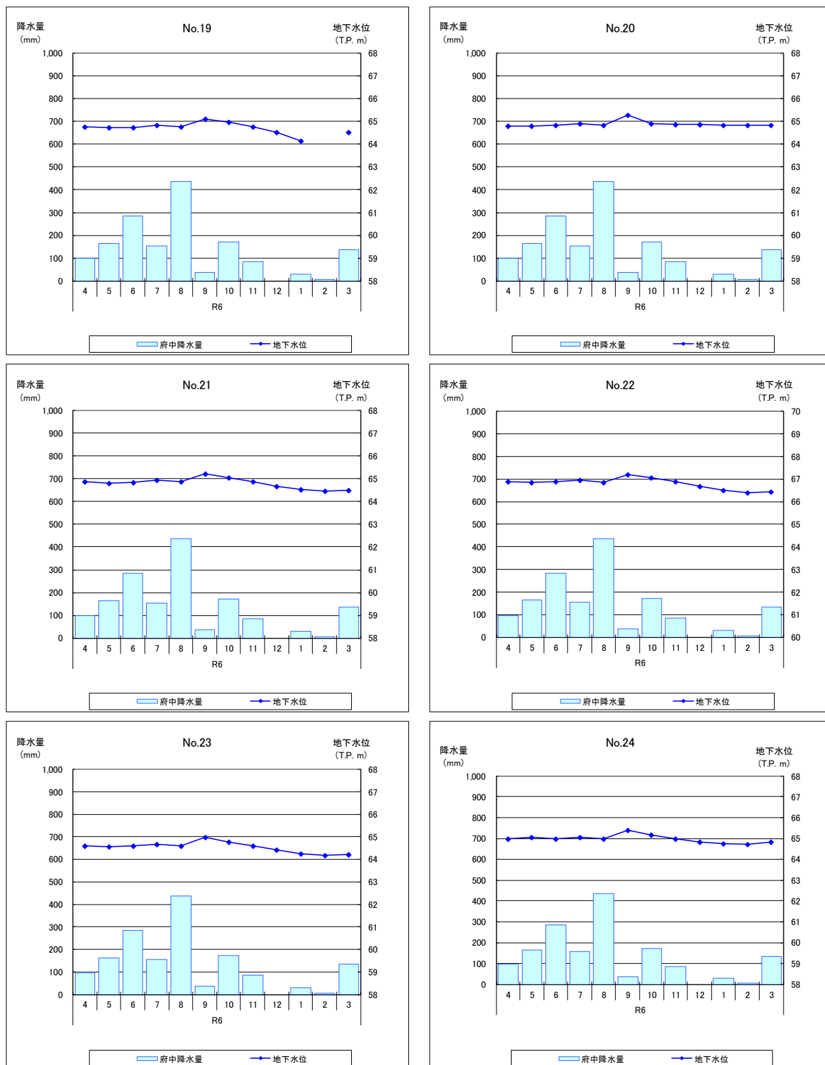
図-3.2(3) 地下水位測定結果及び気象庁府中観測所雨量 (3/6)
