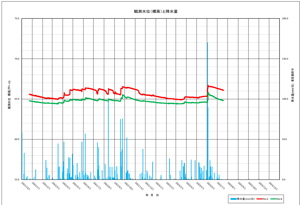
国分寺市新庁舎建設工事 湧水・地下水調査 地下水位観測結果図(No.A、B 標高) (2023/7/19現在)
